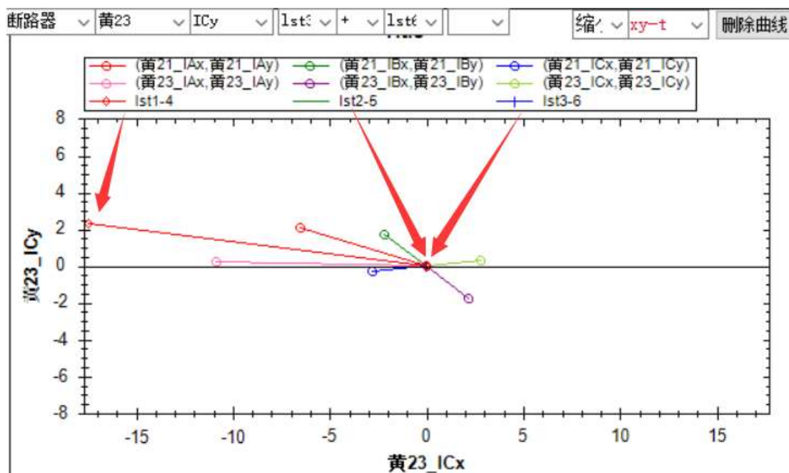
图 7 母线 A 相接地故障情况下黄 21 和黄 23 的三相电流向量，箭头所指分别为故障点的三相电流向量（A 相 Ist1-4，B 相 Ist2-5，C 相 Ist3-6），可见故障点 A 相短路电流很大，B 相、C 相电流为 0。注意和图 6 进行对比验证。
