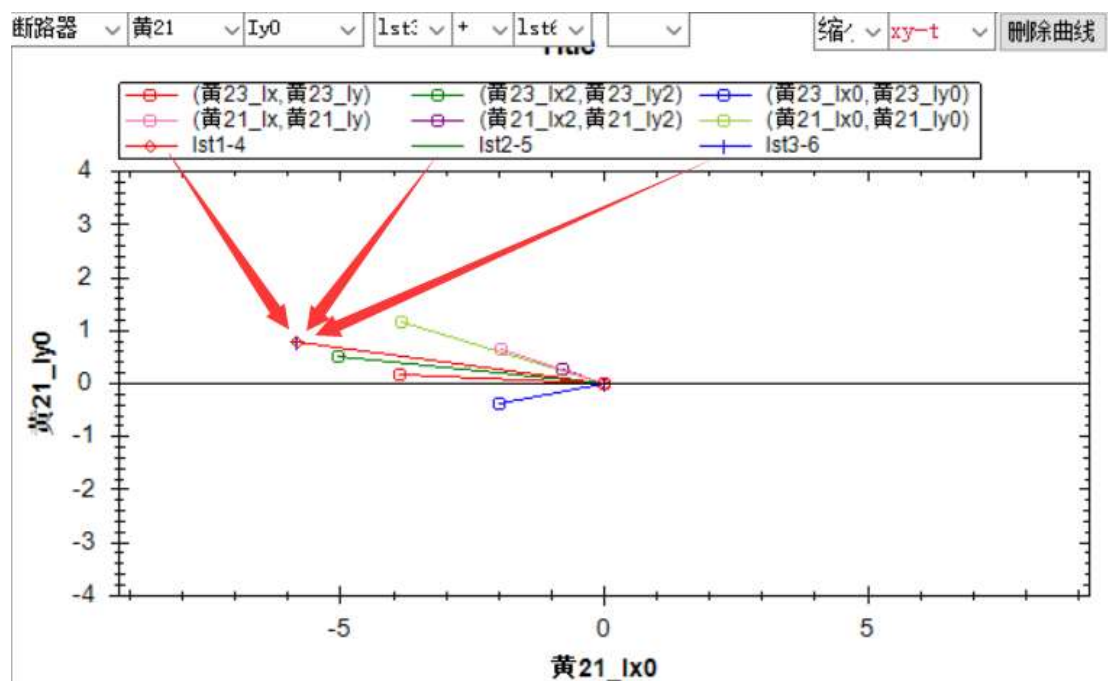
图 6 箭头所指向量分别为故障点的正序、负序、零序电流向量。分别来自黄 23 和黄 21 的正序电流之和、黄 23 和黄 21 的负序电流之和、黄 23 和黄 21 的零序电流之和。
