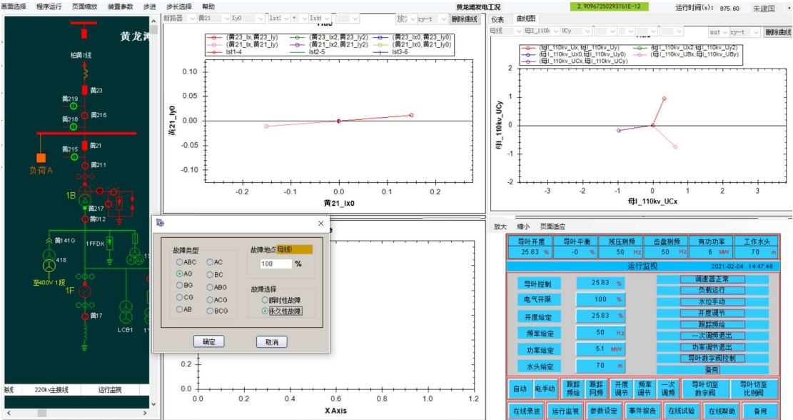
图 4 右键单击母线弹出故障选择对话框，选择“AG”（A相接地故障），“永久故障”。
