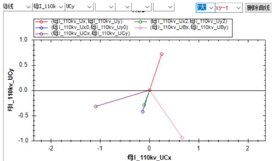
图 8 可见红绿蓝分别为 A 相的正序电压向量、负序电压向量、零序电压向量，合成的 A 相电压向量为 0。B 相电压、C 相电压通过正序负序零序分量可以合成，如图中淡紫和紫色向量所示。
